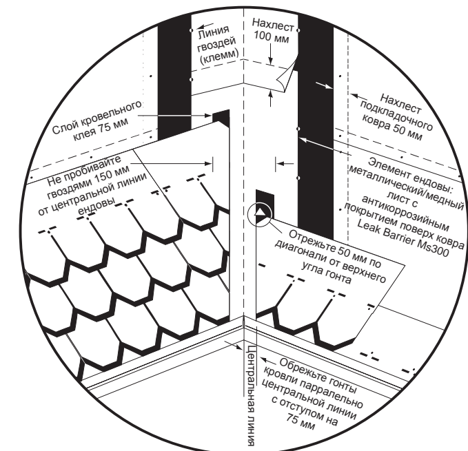
Рисунок 17-11. Устройство ендовы для Carriage House
